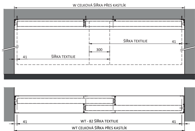
VÍCEHŘÍDELOVÝ SYSTÉM - OD ŠÍŘKY 4,5 m A PRO VYSOKÉ SPUŠTĚNÍ, TYP V1
