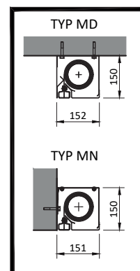
JEDNOHŘÍDELOVÝ SYSTÉM TYPY
