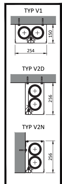
VÍCEHŘÍDELOVÝ SYSTÉM TYPY
