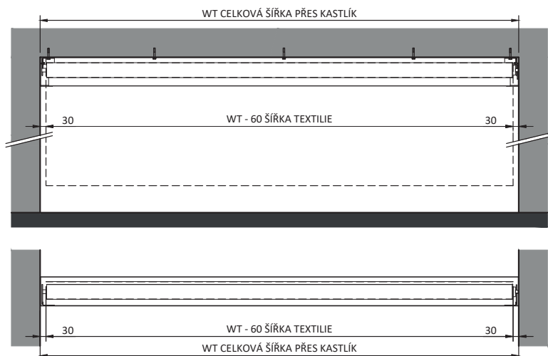
VÍCEHŘÍDELOVÝ SYSTÉM - OD ŠÍŘKY 4,5 m A PRO VYSOKÉ SPUŠTĚNÍ, TYP V1
