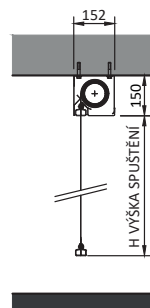
JEDNOHŘÍDELOVÝ SYSTÉM - DO ŠÍŘKY 4,5 m A VÝŠKY SPUŠTĚNÍ DO 4,5 m, TYP MD
