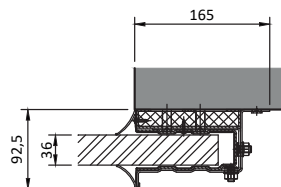
DETAIL VODÍCÍ LIŠTY
