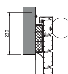
DETAIL NADPRAŽÍ
