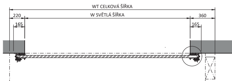
PŮDORYS - UPEVNĚNÍ NA OTVOR
